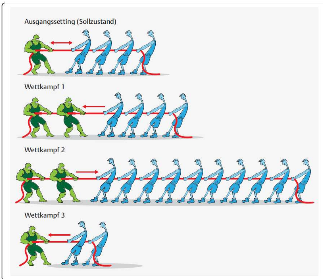
Abb. 8.2 Veranschaulichung der von den Richtwerten (Sollzustand) abweichenden Hormonverhältnisse. Mannschaft A (links) trägt grüne Trikots, Mannschaft B (rechts) blaue. Im Ausgangssetting besteht ein Kräftegleichgewicht, in Wettkampf 1 liegt eine A-Dominanz vor, in Wettkampf 2 eine B-Dominanz und in Wettkampf 3 eine relative A-Dominanz.
